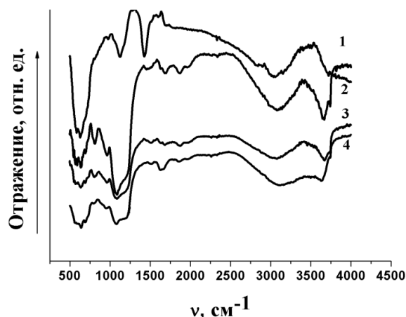
Рис. 3. ІЧ-Фур'є спектри \text{Fe}_3\text{O}_4 (1) та нанокompозитів \text{Fe}_3\text{O}_4/\text{SiO}_2 . Вміст \text{SiO}_2 в нанокompозиті на 1 г \text{Fe}_3\text{O}_4/\text{SiO}_2 – 0,5 г; ПЛ – 0 г (2, варіант 2); 0,7 г (3, варіант 4 а); 0,0007 (4, варіант 4 б).
