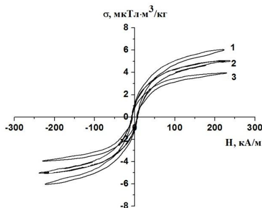
Рис. 4. Петлі гістерезису магнетиту (1) та зразків нанокompозитів \text{Fe}_3\text{O}_4/\text{SiO}_2 (2, 3). Вміст \text{SiO}_2 в нанокompозиті на 1 г \text{Fe}_3\text{O}_4 – 0,5 г; ПЛ – варіант 4 а (2); варіант 4 б (3).
