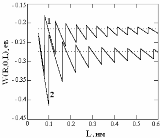
Рис.1. Залежність W(R, 0, L) для зарядів на поверхні півки x = 0 та латеральній відстані між ними R = 0,5 від товщини L РК півки металу з параметрами n = 10^{22} \text{ см}^{-3} та m^* = 0,637 (суцільна крива 1) і n = 5 \cdot 10^{21} \text{ см}^{-3} та m^* = 0,6134 (суцільна крива 2) при \phi = 4,6 еВ. Відповідні пунктирні криві - значення W(R, 0, L \rightarrow \infty) для необмеженого металу.
