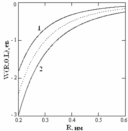
Рис.2. Залежність W(R, 0, L) для зарядів на поверхні ( x = 0 ) РК півки металу з параметрами n = 5 \cdot 10^{21} \text{ см}^{-3} , m^* = 0,6134 та \phi = 4,6 еВ від відстані R між ними для товщин L = d \cdot \omega , коли \omega = 3 (суцільна крива 1) та \omega = 8 (суцільна крива 2) при d = 0,1185 нм. Точкова крива - значення W(R, 0, L \rightarrow \infty) для необмеженого металу.
