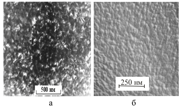
Мал. 3 Мікроструктура плівок а) VB_2 , б) TaB_2
