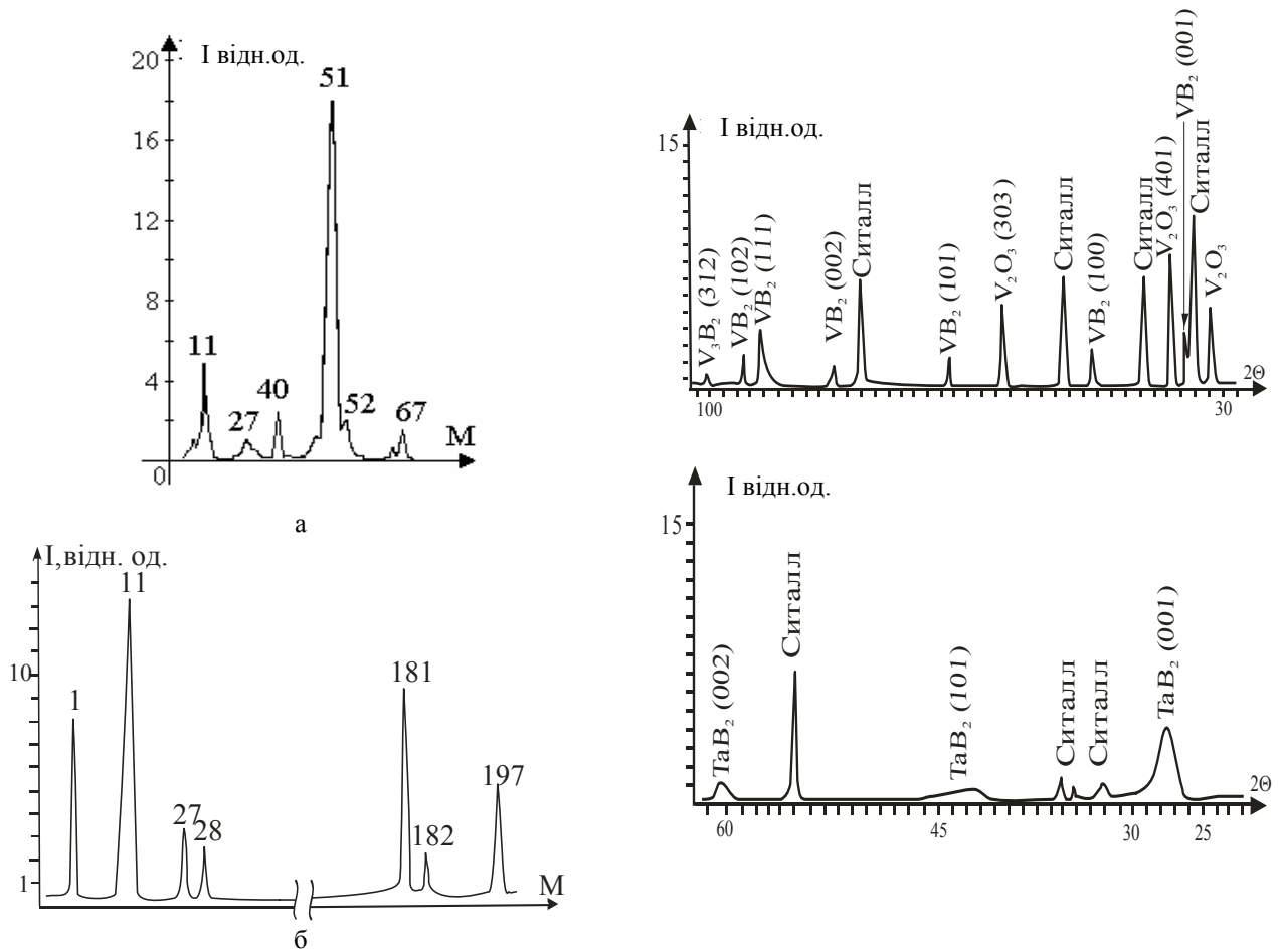
Мал. 1. Мас-спектр а – мішень VB_2 , б – мішень TaB_2 .
