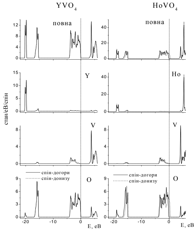
Рис. 2. Повні електронні щільності й повній атомні електронні щільності сполук \text{LnVO}_4 ( \text{Ln}=\text{Y}, \text{Ho} ). Тут і далі на рисунках нуль шкали енергій ( E ) відповідає розрахованому положенню хімічного потенціалу.
