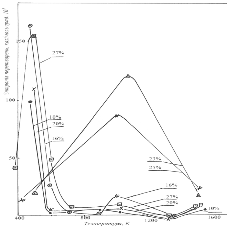
Рис. 6. Температурний хід ентропії перетворення розплавів системи \text{Na}_2\text{O}-\text{B}_2\text{O}_3
