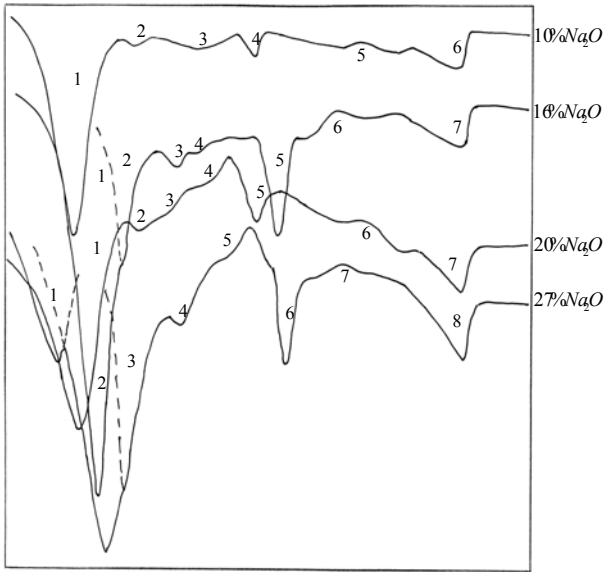
Рис. 3. Дериwатограми складів системи \text{Na}_2\text{O} - \text{B}_2\text{O}_3 (пояснення у тексті)
