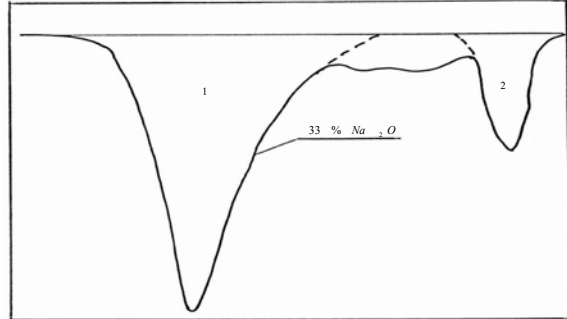
Рис. 5. Дериwатограма складу системи \text{Na}_2\text{O} - \text{B}_2\text{O}_3 (пояснення в тексті)
