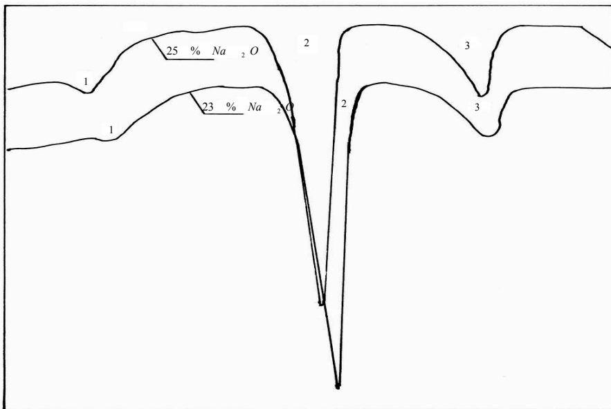
Рис. 4. Дериwатограми складів системи \text{Na}_2\text{O} - \text{B}_2\text{O}_3 (пояснення у тексті).
