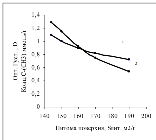
Рис. 8. Залежність концентрації метильних груп S_{\text{спт.}} (C_{\text{СН}_3}) (1) та оптичної густини D (2) від питомої поверхні S_{\text{спт.}} кремнезему марки АМС.
