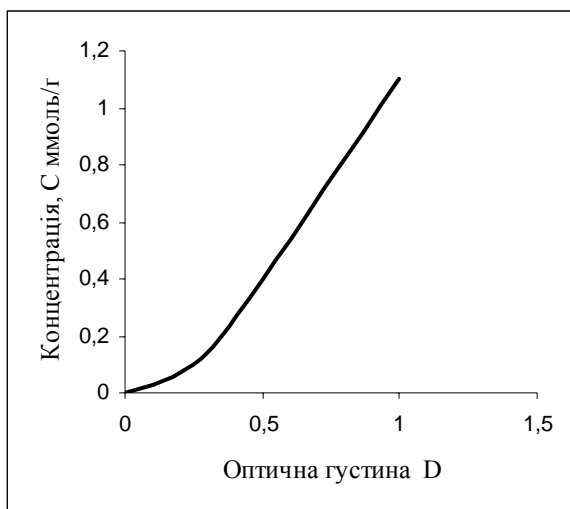
Рис. 1. Залежність концентрації метильних груп ( C_{CH_3} ) в MAS-200 від оптичної густини D .
