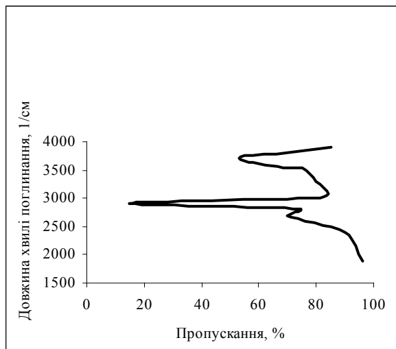
Рис. 2. ІЧ-спектр пірогенного кремнезему марки MAS-200.
