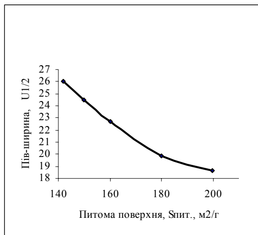
Рис. 7. Залежність півширини U_{1/2} від питомої поверхні для кремнезему марки АМС.
