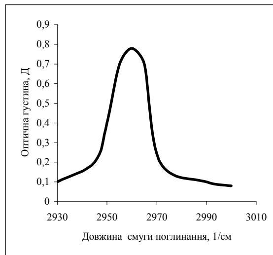
Рис. 10. Залежність оптичної густини ( D ) від довжини хвилі поглинання ( 1/\lambda ) для кремнезему марки АМС-200.
