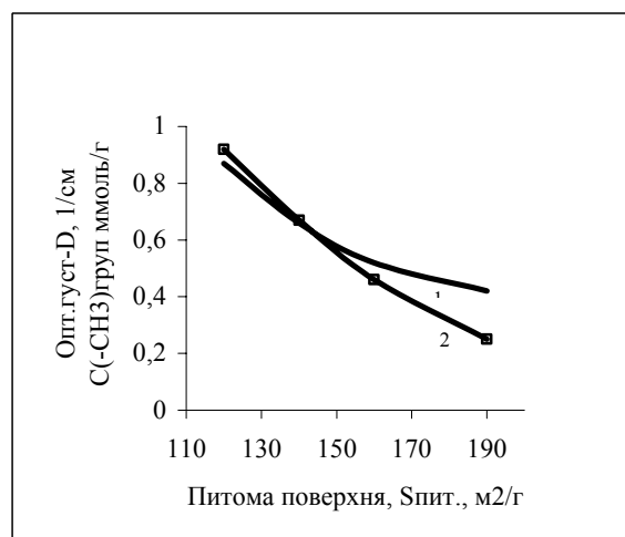
Рис. 4. Залежність концентрації метильних груп (1) ( C_{CH_3} ) та оптичної густини (2) від питомої поверхні для MAS-200 ( S_{пит.} ).
