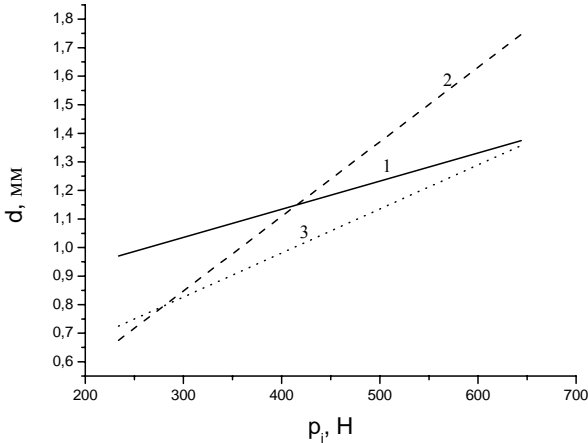
Рис. 1. Залежність діаметра плями зносу (d) сталі ШХ-15 від навантаження на одну кульку ( p_i ) в середовищі мастильних матеріалів на основі ПФПЕ: 1 – ПЕФ-130/110; 2 – ПЕФ-130/110 + активний яскраво-блакитний 5“3”Ш (48%); 3 – ПЕФ-130/110 + активний яскраво-блакитний 5“3”Ш (20 %).
