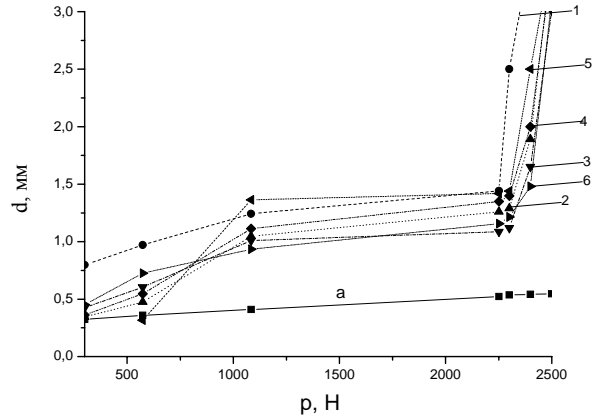
Рис. 2. Залежність плями зносу (d) сталі ШХ-15 від осьового навантаження (p) в середовищі мастильних матеріалів: 1 – ПЕФ-130/110 (●); 2 – ПЕФ-130/110 + I (▲); 3 – ПЕФ-130/110 + II (▼); 4 – ПЕФ-130/110 + III (◆); 5 – ПЕФ-130/110 + IV (◀); 6 – ПЕФ-130/110 + V (▶), а – лінія діаметрів пружної деформації за Герцем.
