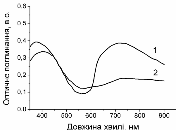
Рис. 3. Зміна спектрів пропускання при різних напругах на двох електродному оптичному елементі: U = +1V(1) ; U = -1V(2)
