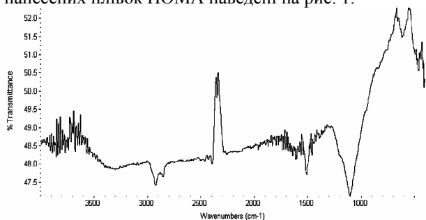
Рис. 1. Інфрачервоні спектри ПОМА з використанням Фур'є-перетворення
